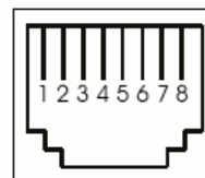
Az RJ-45 csatlakozó lábkiosztása
